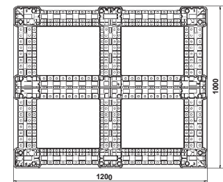
底視圖
