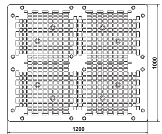
頂視圖
