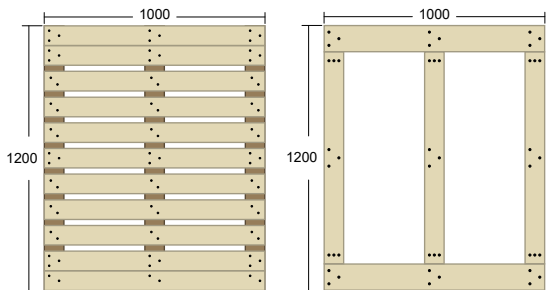
俯視圖
