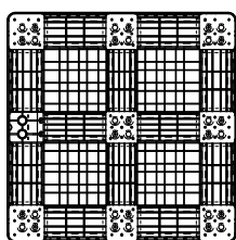
底視圖
